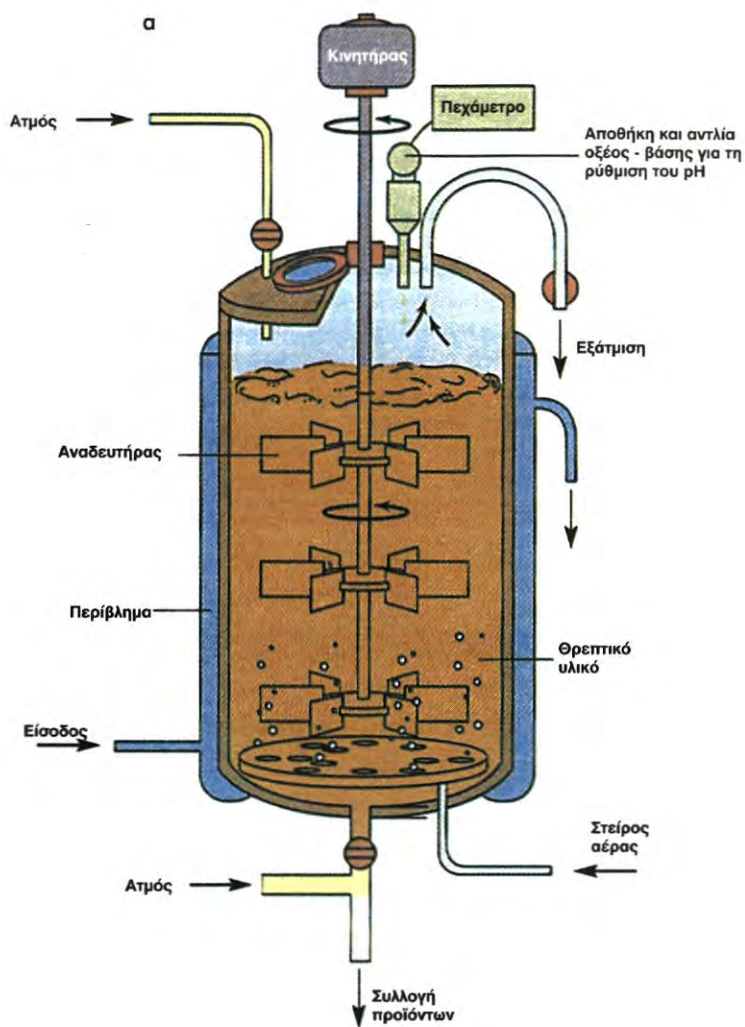
Εικόνα 7.3 α. Διαγραμματική απεικόνιση βιοαντιδραστήρα, όπου φαίνονται τα διάφορα τμήματά του, καθώς και οι συσκευές ελέγχου των συνθηκών ζύμωσης β. Φωτογραφία βιοαντιδραστήρα.
