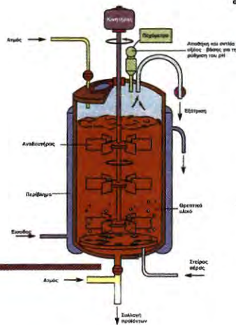
Εικόνα 7.3α Διαγράμμιση σπειρώσεως βιοανθρακίστη, όπου φαίνονται τα διάφορα τμήματά του, καθώς και οι συσκευές ελέγχου των συνθηκών ζύμωσης β. Φωτογραφία βιοεπιχείρησης.
