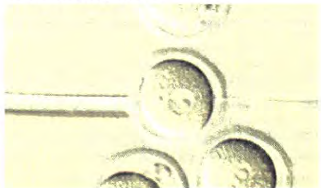
Εικόνα 9.6 Μικροέγχυση DNA.
