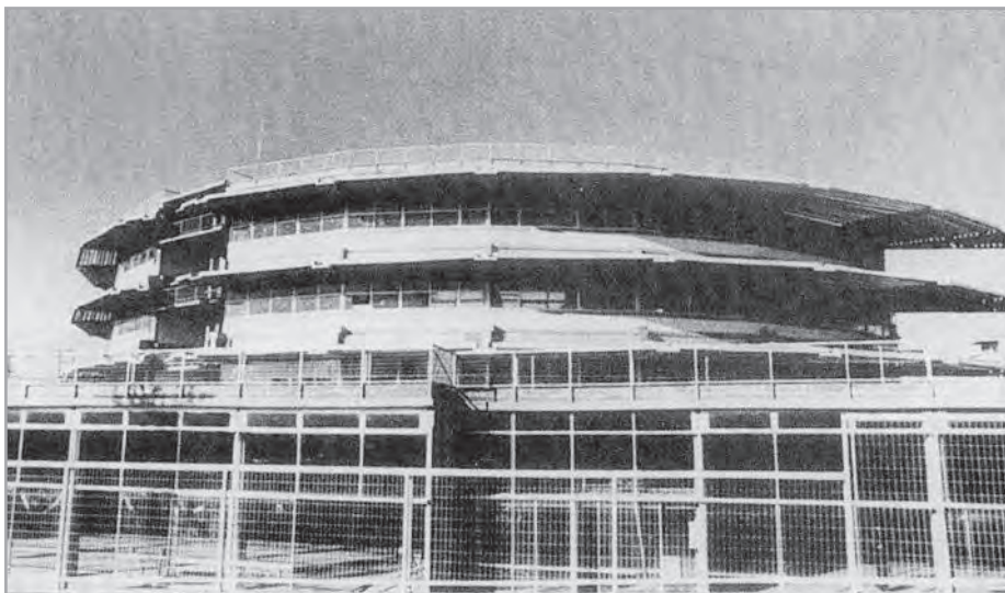
Τάκης Ζενέτος (1926-1977), Γυμνάσιο και Λύκειο, 1970-76, Άγιος Δημήτριος, Αθήνα. Ο καιρ'εξοχίν αρχιτέκτονας του ελληνικού μοντερνισμού, ανατρέπει με το κτήριο αυτό το καθιερωμένο μοντέλο ανάπτυξης του σχολικού χώρου. Με τη βοήθεια της τεχνολογίας και των σύγχρονων υλικών (μπετόν, μέταλλο και γυαλί) ξεπερνά το παραλληλεπίπεδο σχήμα των μοντέρνων κατασκευών, δημιουργώντας ένα κυκλικό κτήριο με ανοικτούς, ευέλικτους χώρους και πολλές δυνατότητες χρήσης και εφαρμογής των πρακτικών του σύγχρονου σχολείου.
