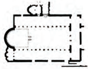
Κάτοψη της βασιλικής της Αχειροποιήτου στη Θεσσαλονίκη (5ος-6ος αι.). Είναι ο πιο χαρακτηριστικός αρχιτεκτονικός τύπος εκκλησίας της παλαιοχριστιανικής εποχής. Έχει πρόναο και χωρίζεται σε τρία κλίτη.
