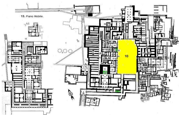
κάτοψη μινωικού ανακτόρου
