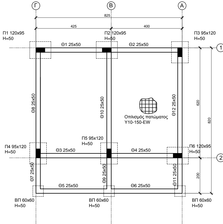
ΞΥΛΟΤΥΠΟΣ ΘΕΜΕΛΙΩΣΗΣ ΚΛ. 1:100
