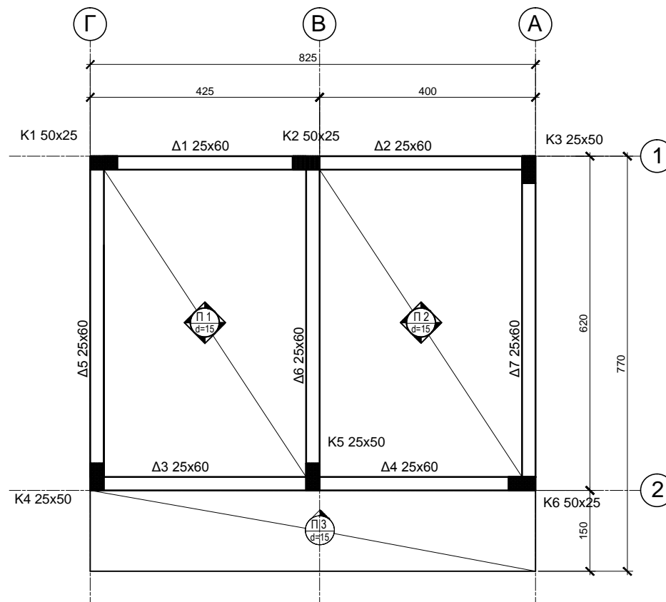
ΞΥΛΟΤΥΠΟΣ ΠΛΑΚΑΣ ΟΡΟΦΗΣ ΚΛ. 1:100
