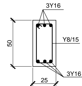
ΤΟΜΗ ΘΕΜΕΛΙΟΔΟΚΟΥ ΚΛ. 1:25
