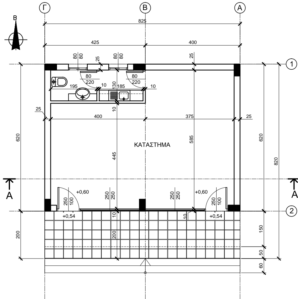
ΚΑΤΟΨΗ ΙΣΟΓΕΙΟΥ
