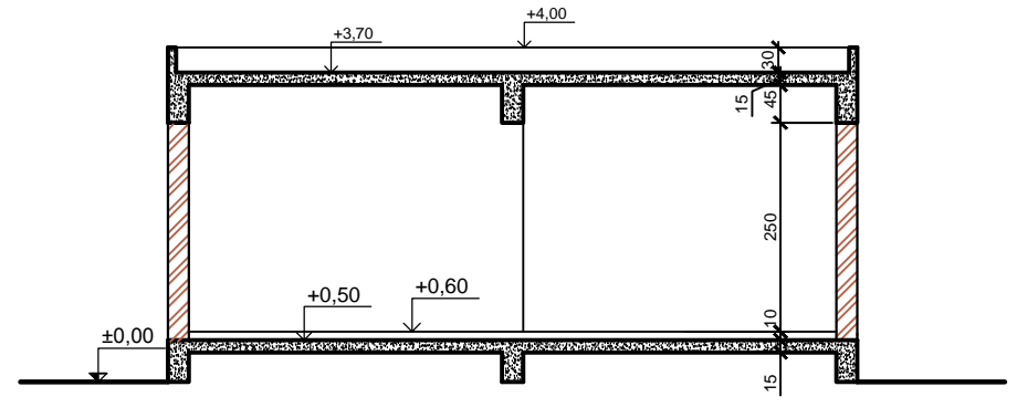
ΤΟΜΗ Α-Α
