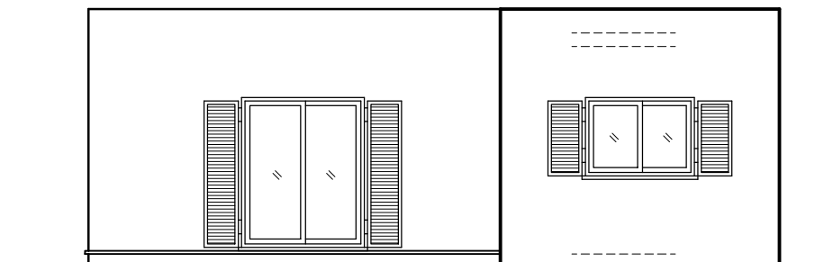
ΠΙΣΩ ΟΨΗ (ΝΟΤΙΑ ΟΨΗ) ΚΛΙΜΑΚΑ 1:100
