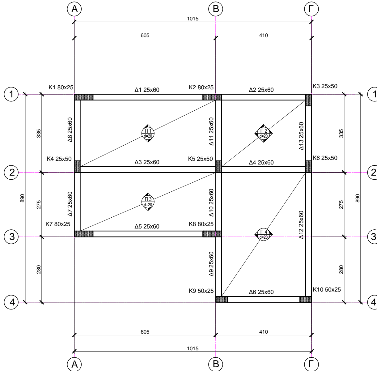
ΚΑΤΟΨΗ ΕΥΛΟΤΥΠΟΥ ΠΛΑΚΑΣ ΟΡΟΦΗΣ ΚΛΙΜΑΚΑ 1:100
