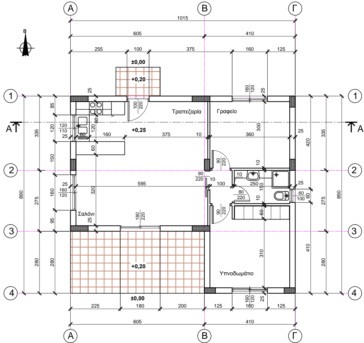
ΚΑΤΟΨΗ ΙΣΟΓΕΙΟΥ ΚΛΙΜΑΚΑ 1:100
