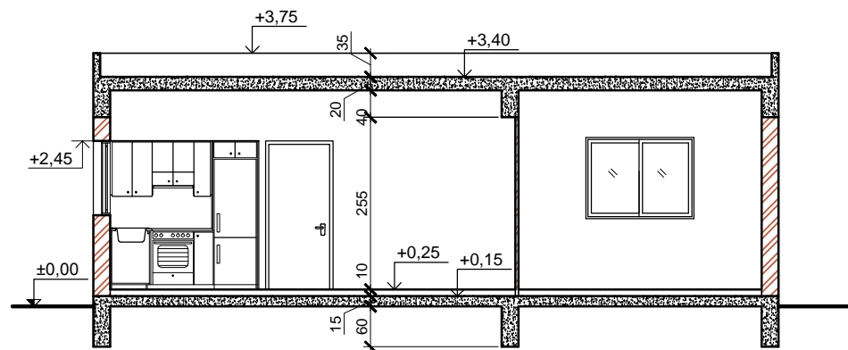
ΤΟΜΗ Α-Α ΚΛΙΜΑΚΑ 1:100
