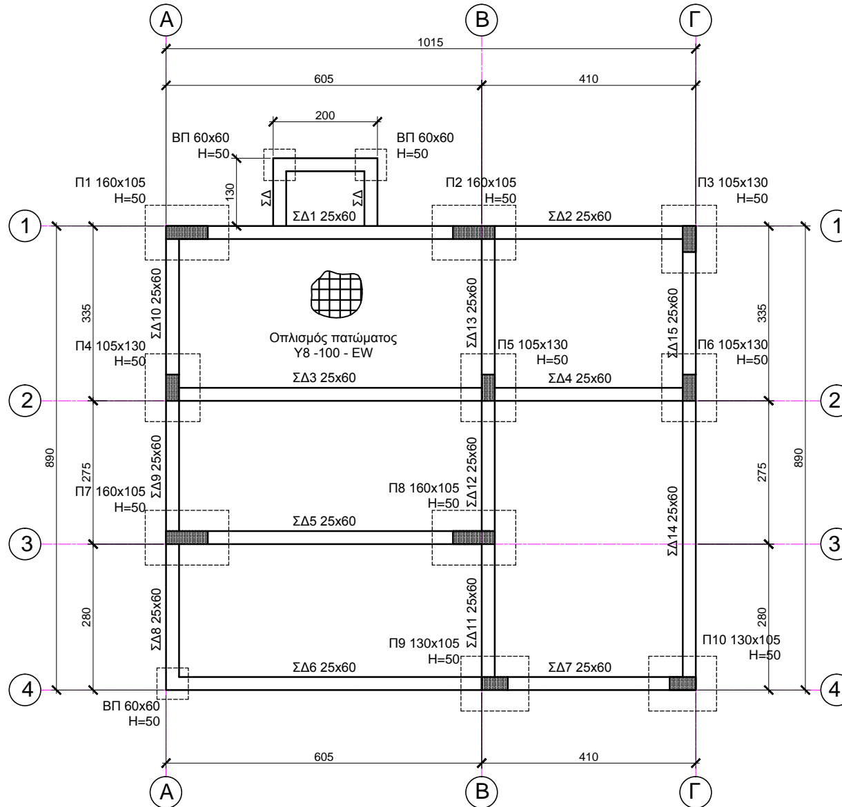
ΚΑΤΟΨΗ ΕΥΛΟΤΥΠΟΥ ΘΕΜΕΛΙΩΣΗΣ ΚΛΙΜΑΚΑ 1:100
