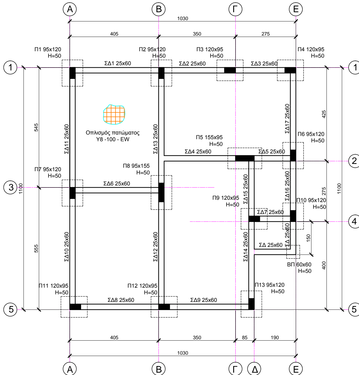
ΚΑΤΟΨΗ ΕΥΛΟΤΥΠΟΥ ΘΕΜΕΛΙΩΣΗΣ ΚΛΙΜΑΚΑ 1:100
