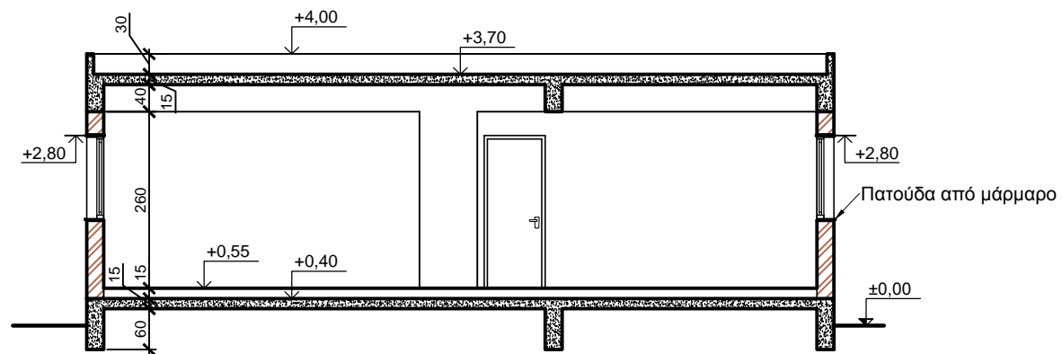
ΤΟΜΗ Α-Α ΚΛΙΜΑΚΑ 1:100
