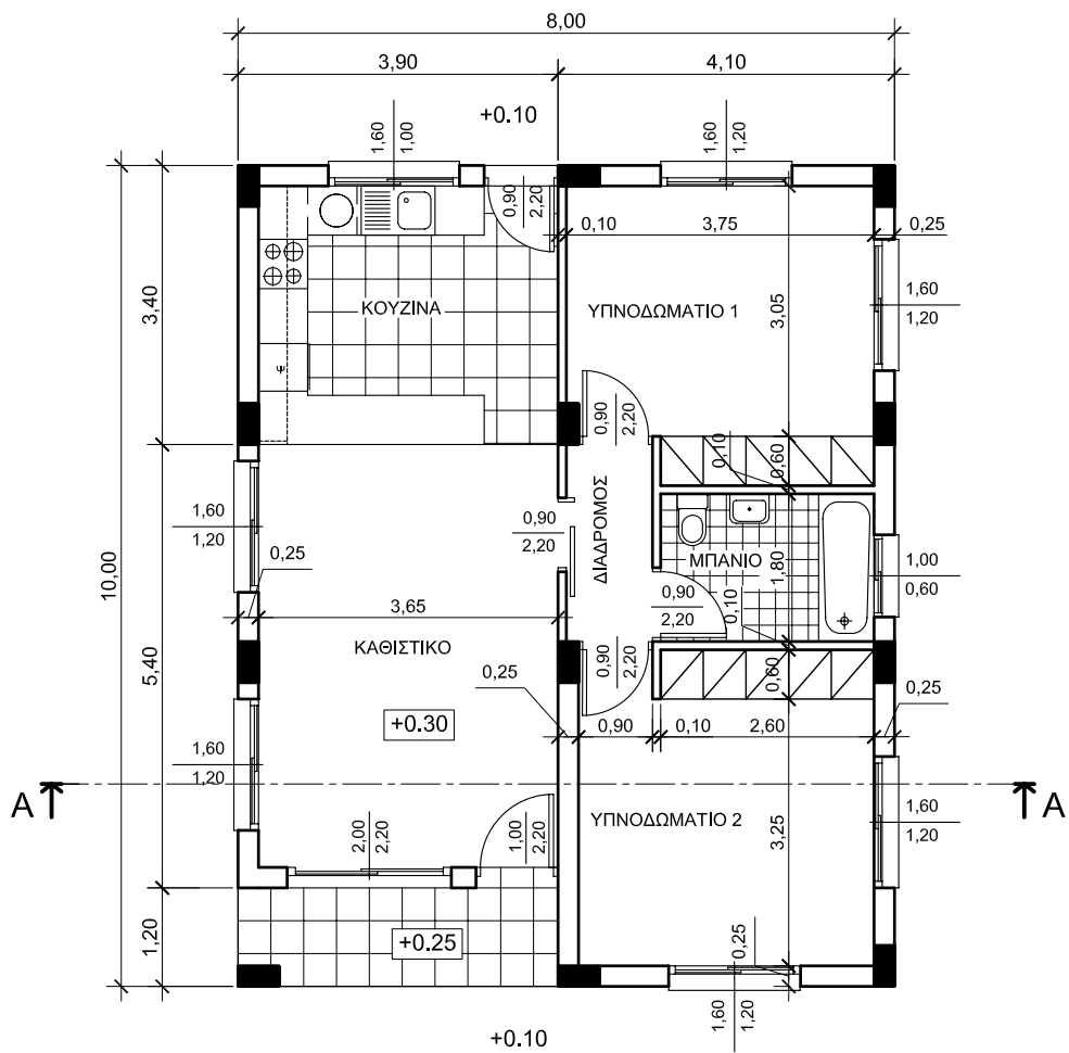
ΚΑΤΟΨΗ ΙΣΟΓΕΙΟΥ ΚΛ. 1:100
