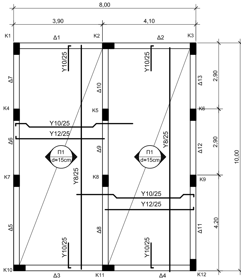
ΚΑΤΟΨΗ ΞΥΛΟΤΥΠΟΥ ΠΛΑΚΑΣ ΚΛ. 1:100
