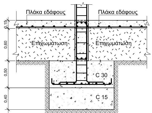
ΤΟΜΗ ΠΕΔΙΛΟΥ Κ5 ΕΚΤΟΣ ΚΛΙΜΑΚΑΣ
