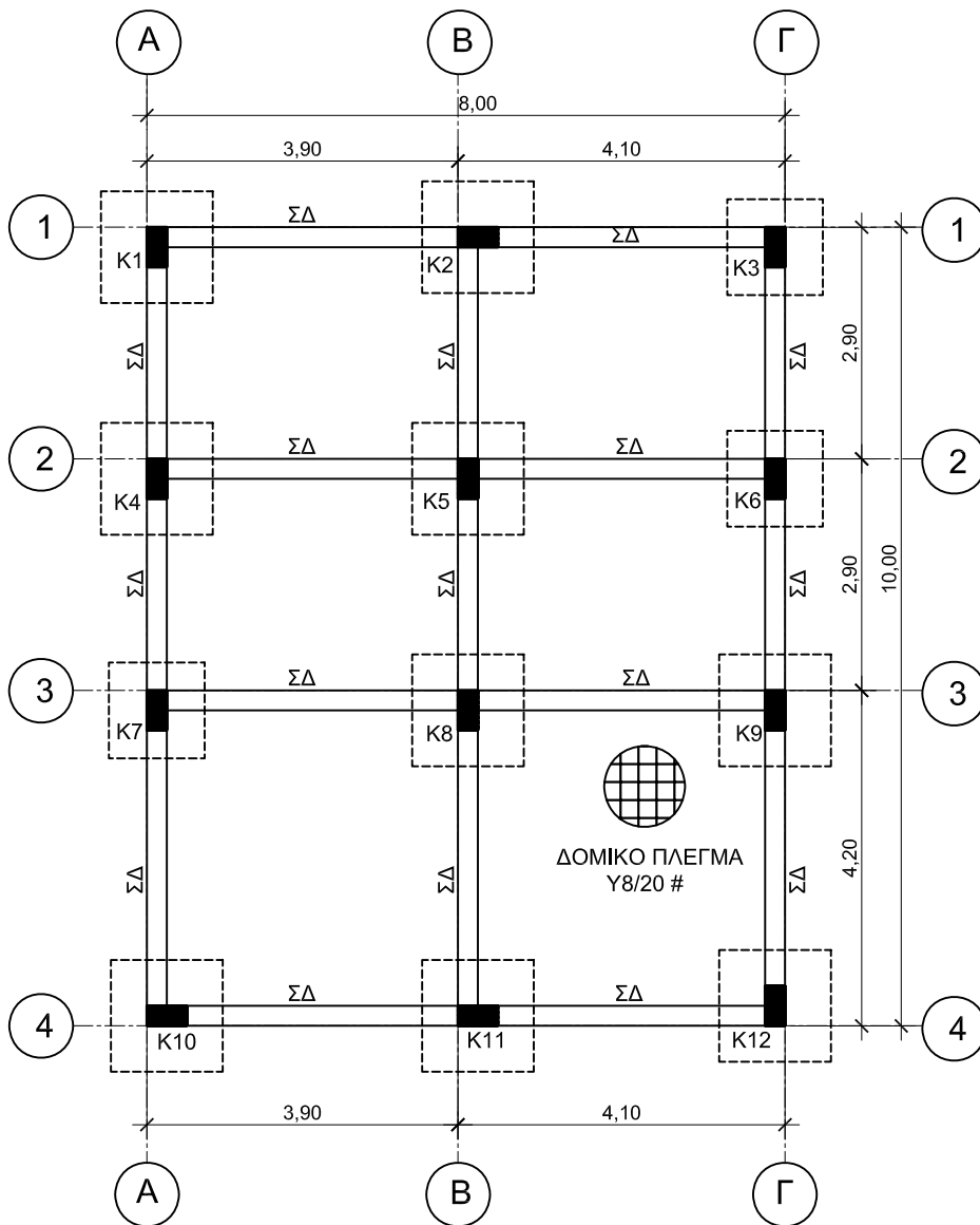
ΚΑΤΟΨΗ ΘΕΜΕΛΙΩΝ ΚΛ. 1:100
