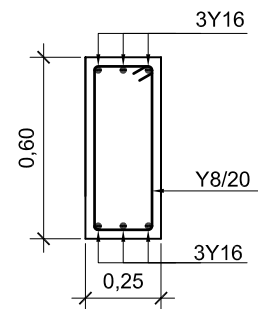
ΤΟΜΗ ΣΥΝΔΕΤΗΡΙΑΣ ΔΟΚΟΥ ΣΔ ΚΛ. 1:25
