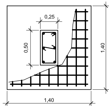
ΤΟΜΗ ΠΕΔΙΛΟΥ Κ5 ΕΚΤΟΣ ΚΛΙΜΑΚΑΣ
