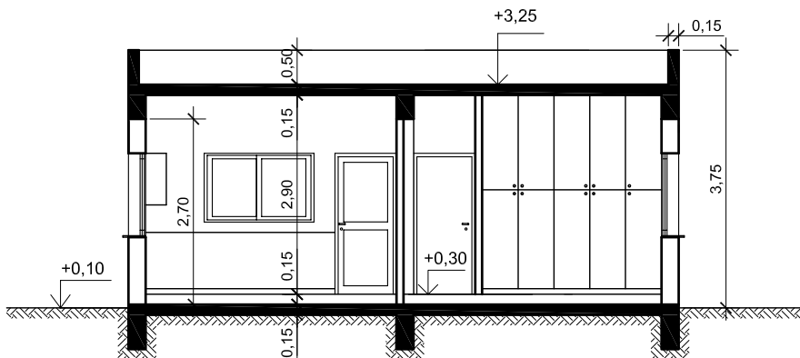
ΤΟΜΗ Α-Α ΚΛ. 1:100
