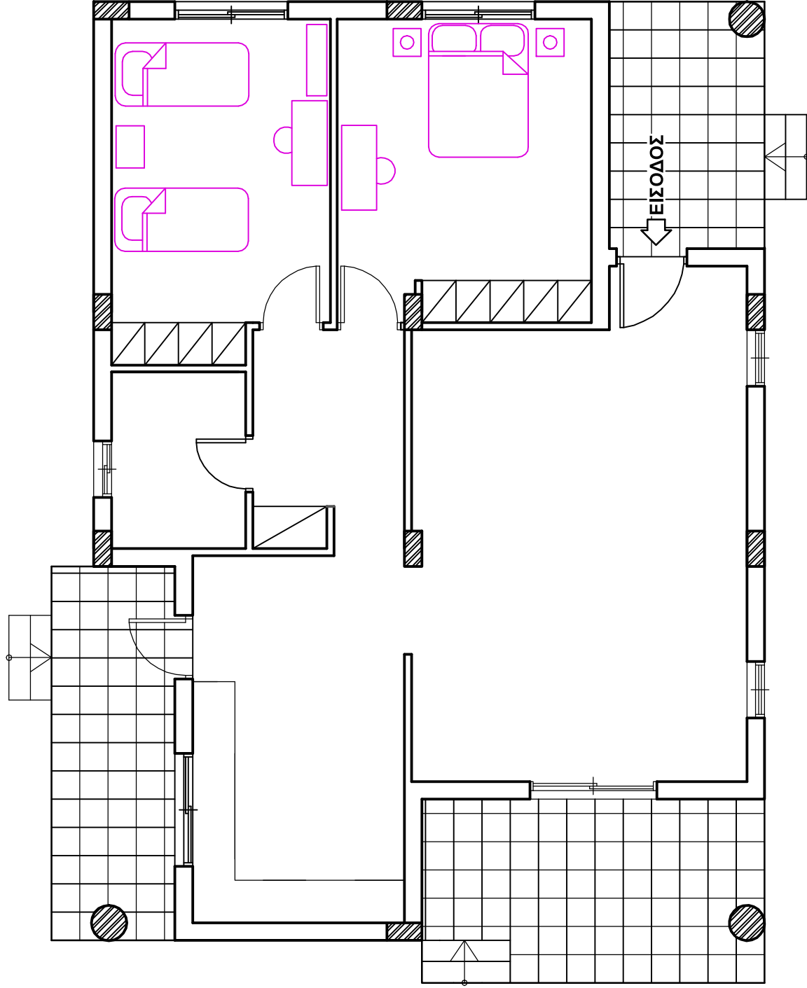
Κάτωψη Κατοικίας ΚΛΙΜΑΚΑ 1:50
