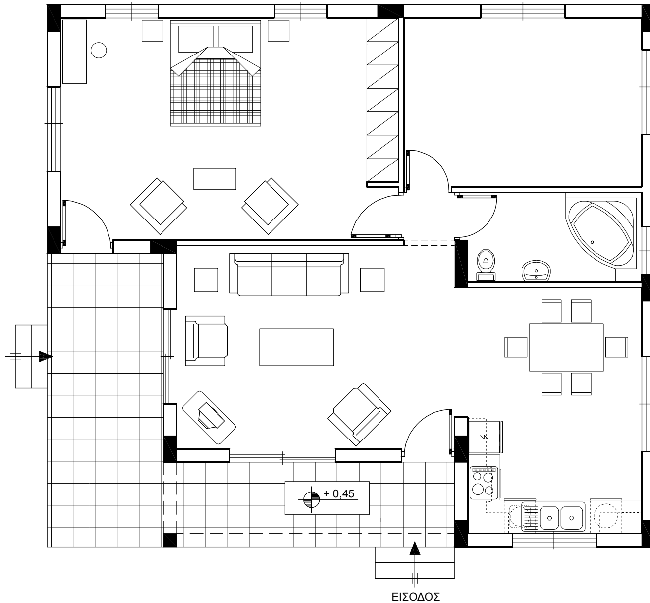
ΚΑΤΟΨΗ ΚΛ. 1:50
