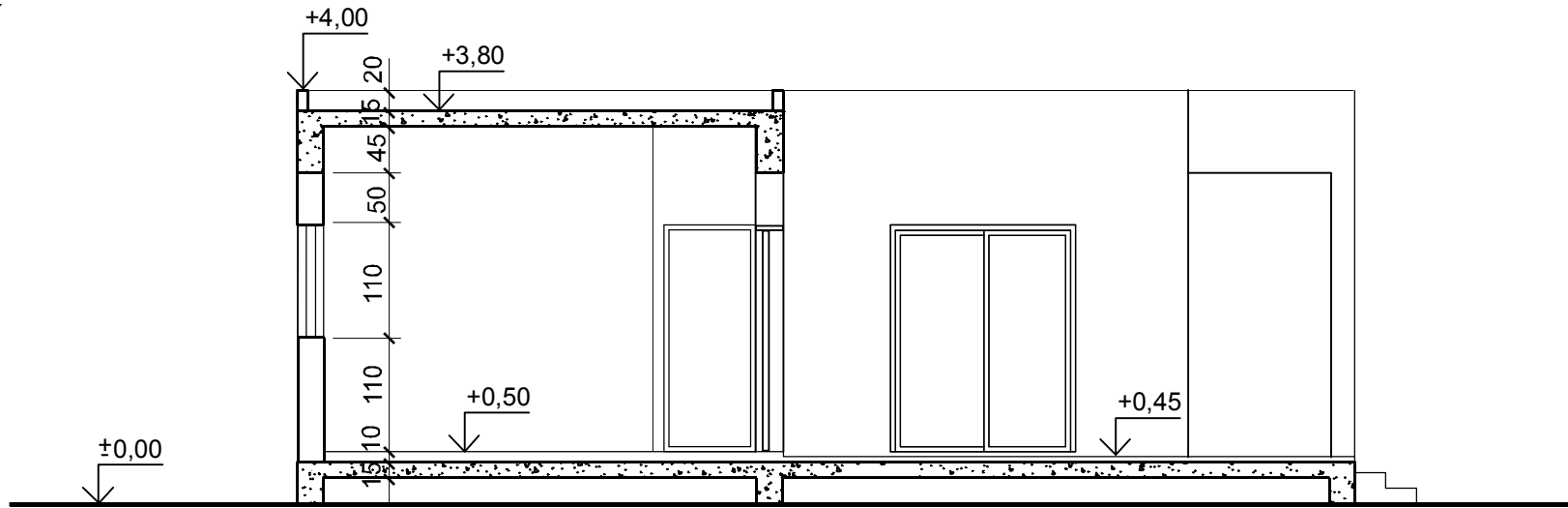
ΤΟΜΗ Α-Α ΚΛ. 1:50
