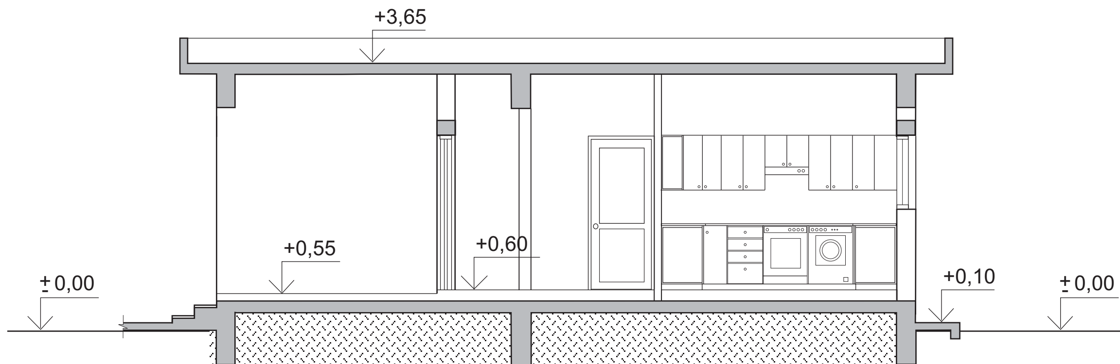
ΤΟΜΗ Β-Β ΚΛ. 1:50
