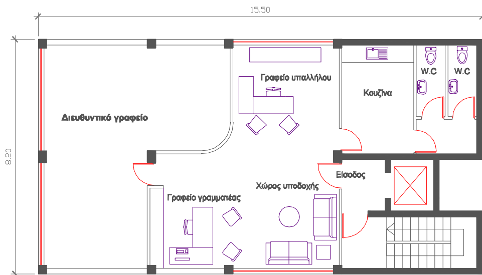
ΚΑΤΟΨΗ ΓΡΑΦΕΙΩΝ ΚΛΙΜΑΚΑ 1:100
