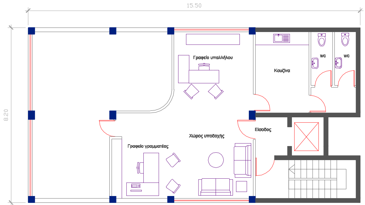
ΚΑΤΩΦΗ ΓΡΑΦΕΙΩΝ ΚΛΙΜΑΚΑ 1:50
