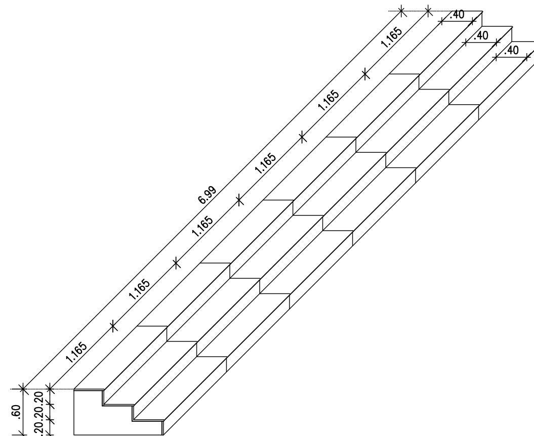
ΙΣΟΜΕΤΡΙΚΟ ΚΛΙΜΑΚΩΤΟΥ ΒΑΘΡΟΥ ΜΟΥΣΙΚΗΣ ΚΛΙΜΑΚΑ: 1:50
