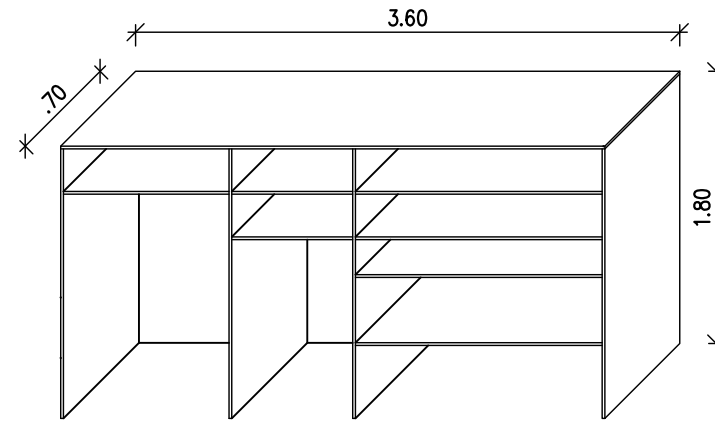
ΙΣΟΜΕΤΡΙΚΟ ΡΑΦΙΩΝ ΜΟΥΣΙΚΩΝ ΟΡΓΑΝΩΝ -Α- ΚΛΙΜΑΚΑ: 1:50
