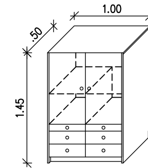
ΙΣΟΜΕΤΡΙΚΟ ΕΠΙΠΛΟΥ ΓΙΑ ΣΤΕΡΕΟΦΩΝΙΚΟ ΣΥΣΤΗΜΑ ΚΛΙΜΑΚΑ: 1:50
