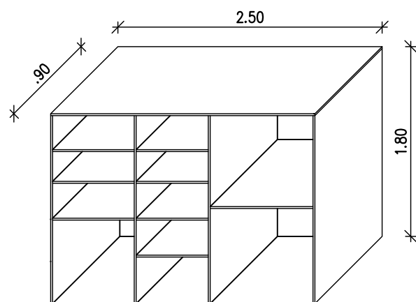
ΙΣΟΜΕΤΡΙΚΟ ΡΑΦΙΩΝ ΜΟΥΣΙΚΩΝ ΟΡΓΑΝΩΝ -Β- ΚΛΙΜΑΚΑ: 1:50
