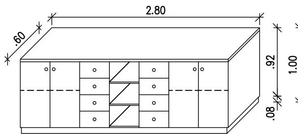
ΙΣΟΜΕΤΡΙΚΟ ΕΠΙΠΛΟΥ ΧΑΜΗΛΟΥ -Γ- ΚΛΙΜΑΚΑ: 1:50
