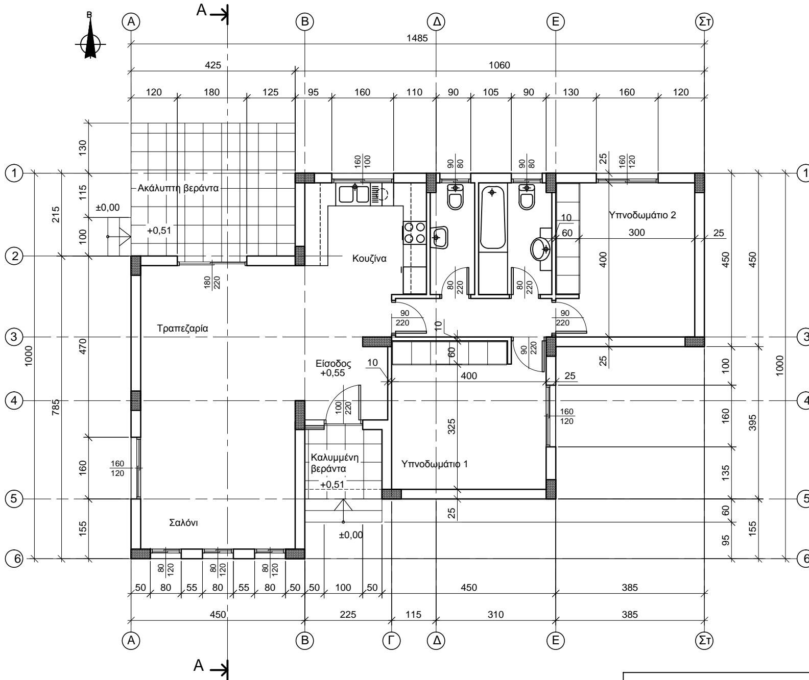
ΚΑΤΟΨΗ ΙΣΟΓΕΙΟΥ ΚΛ. 1:100
