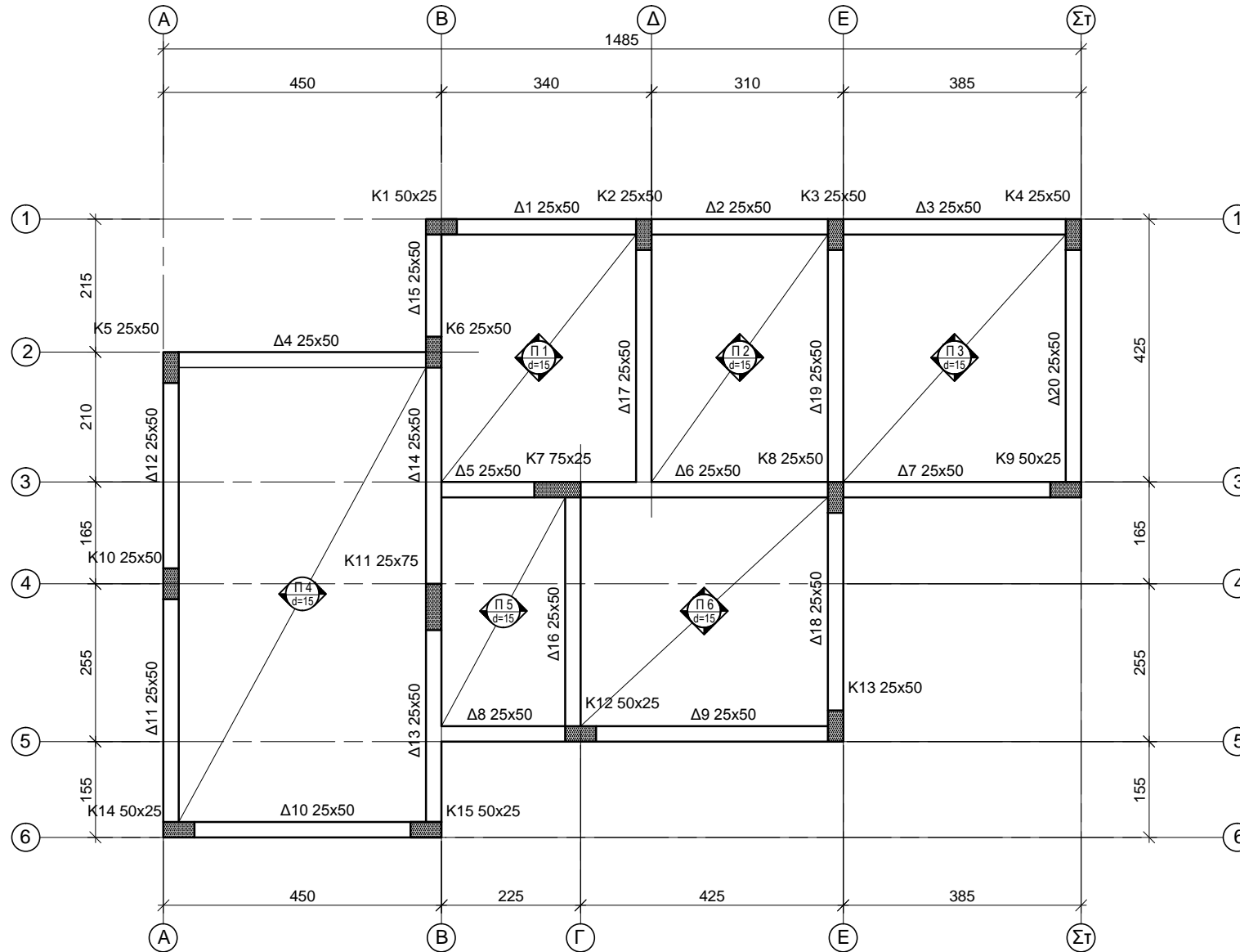
ΕΥΛΟΤΥΠΟΣ ΠΛΑΚΑΣ ΟΡΟΦΗΣ ΚΛ. 1:100
