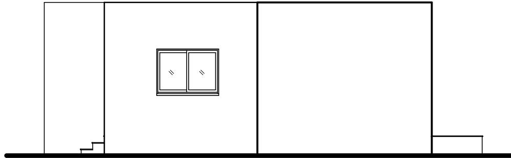
ΠΛΑΓΙΑ ΟΨΗ (ΑΝΑΤΟΛΙΚΗ) ΚΛ. 1:100
