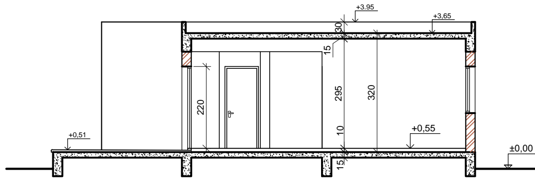
TOMH A - A ΚΛ. 1:100
