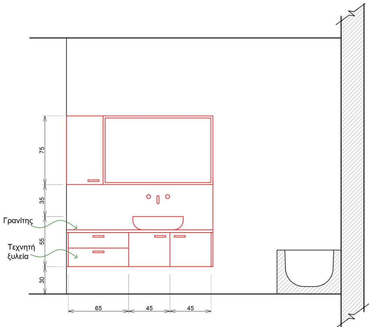
ΟΨΗ Α-Α ΚΛΙΜΑΚΑ 1:25
