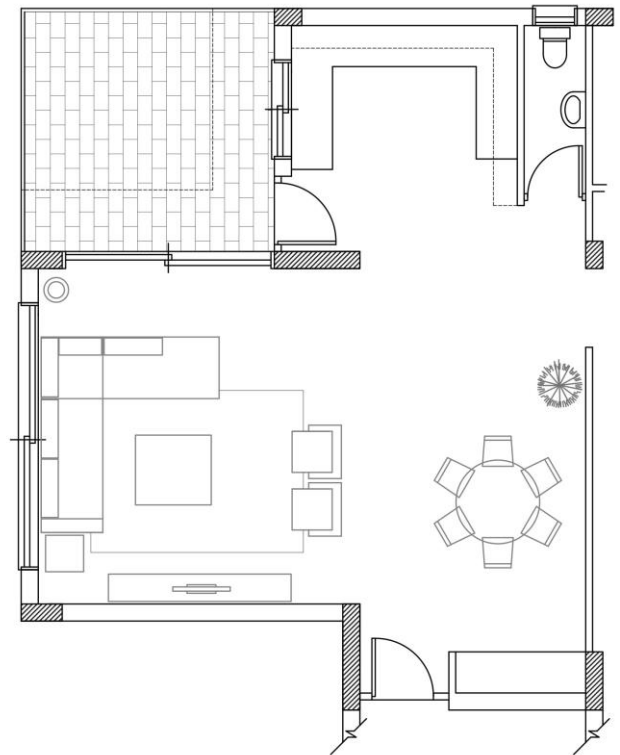
ΚΑΤΩΗ ΚΑΘΙΣΤΙΚΟΥ - ΤΡΑΠΕΖΑΡΙΑΣ ΚΛΙΜΑΚΑ 1:50
