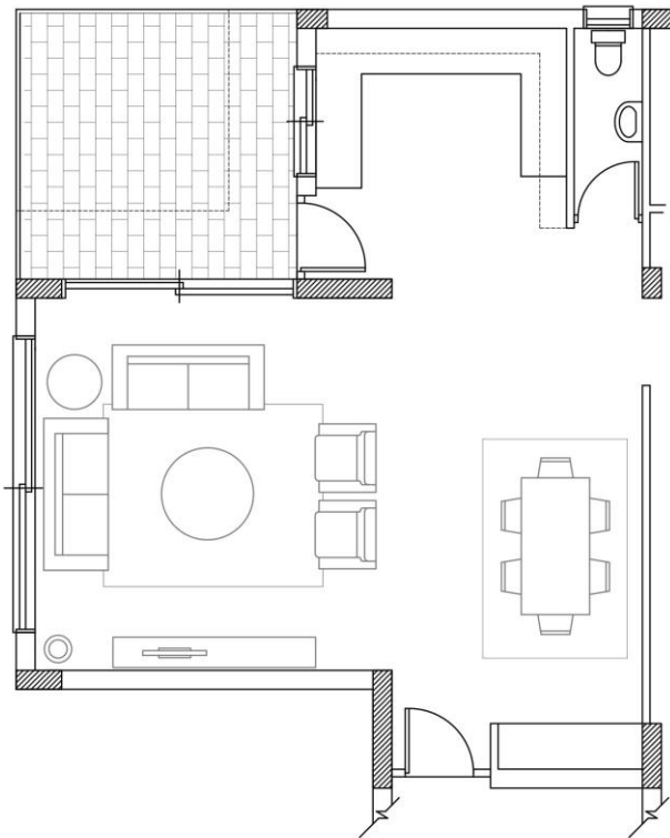
ΚΑΤΩΗ ΚΑΘΙΣΤΙΚΟΥ - ΤΡΑΠΕΖΑΡΙΑΣ ΚΛΙΜΑΚΑ 1:50
