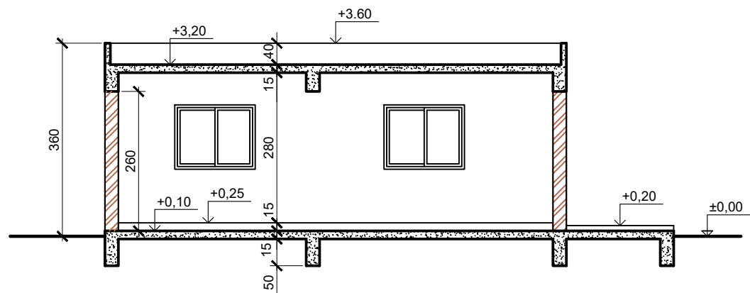
ΤΟΜΗ Α - Α ΚΛ. 1:100
